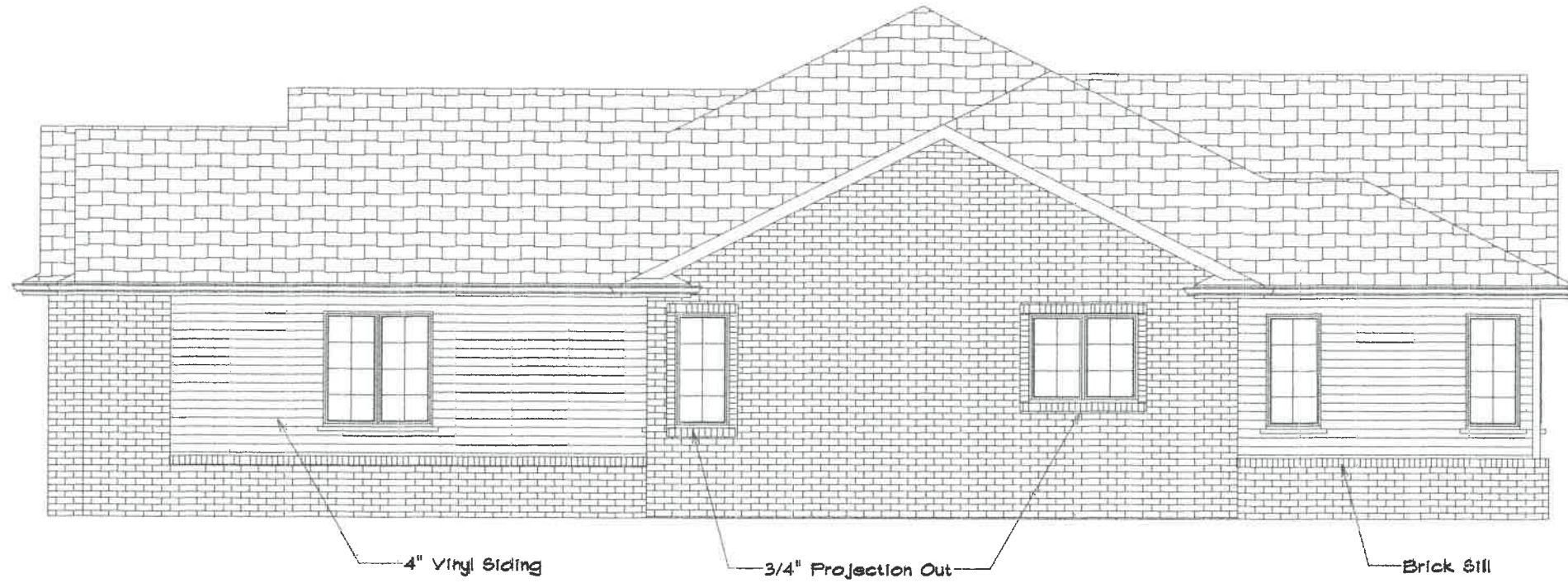
RIGHT ELEVATION Condo 1106
